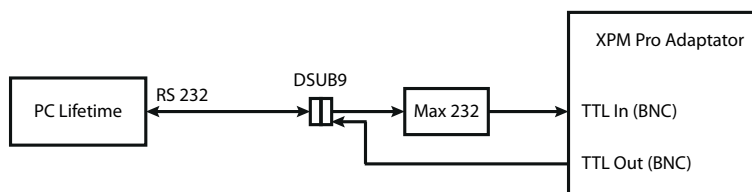
Figure E.2 – Schéma de la connexion de handshaking . Le port série (RS232) du PC Lifetime est relié aux bornes TTL In et TTL Out du boîtier XPMPro Adaptator par l'intermédiaire d'un circuit intégré dans le sens Lifetime vers AFM, et par un simple câble dans l'autre sens.
