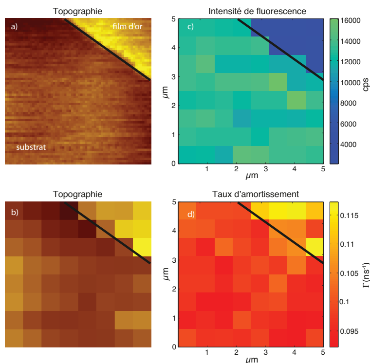
Figure 4.15 – a) Image AFM (topographie) d'une zone de 5 \mu\text{m} de côté constituée d'un film d'or (15 nm d'épaisseur, quasi-continu) sur un substrat de verre. b) même image que a) avec 8 points au lieu de 64. c) Intensité de fluorescence d'une source (centre NV dans un nanodiamant) balayée en champ proche de b). d) Taux d'amortissement de la source fluorescente à sur la zone b). Les images b), c) et d) ont été acquises pendant le même balayage.
